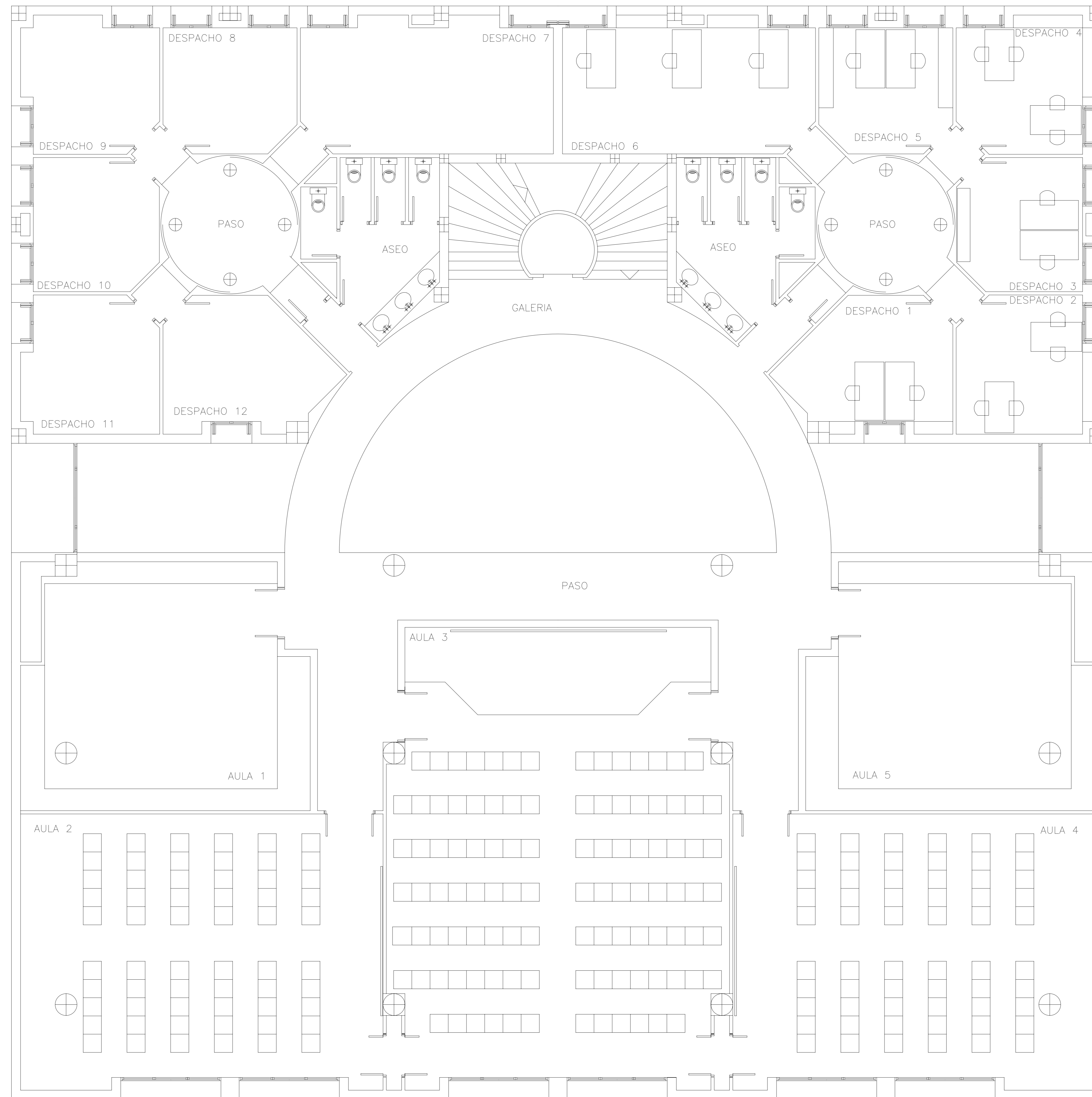
PLANTA PRIMERA ALBANILERIA
